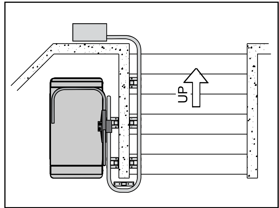
rechte trap met parkeerruimte voor het platform
