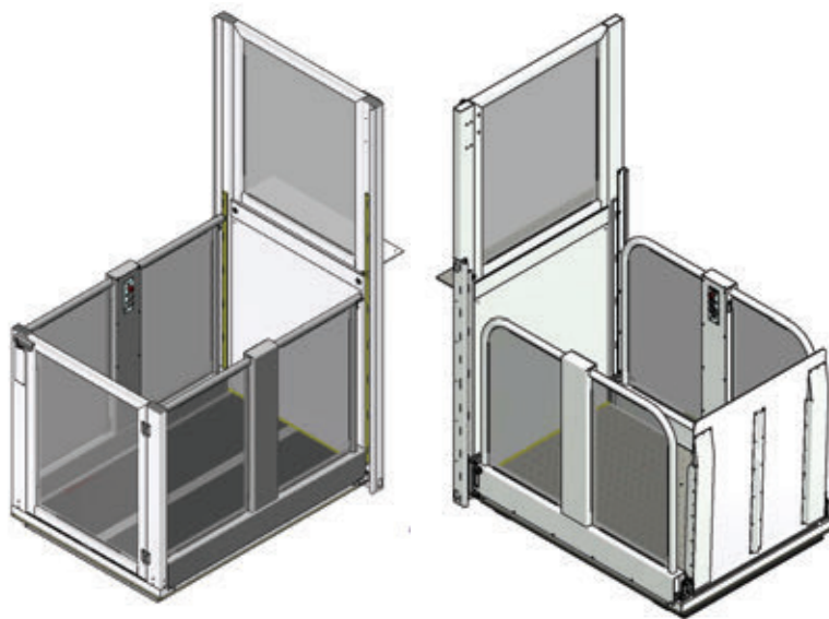
Schematische tekening van uitvoeringen met de deur en oprit op het platform
