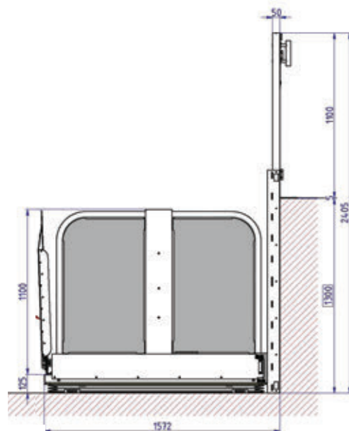
Voorbeeld bouwtekening
